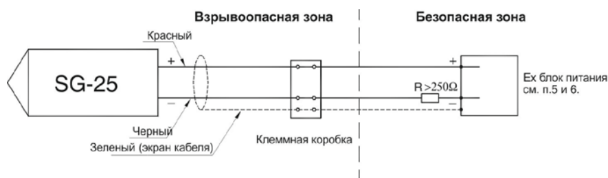
Рисунок 5 – Схема электрических подключений преобразователей модификаций PC-SG-25, PC-SG-25S с выходным сигналом от 4 до 20 мА в Ex исполнении
