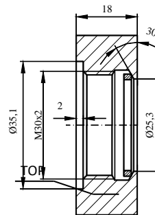
Рисунок Д.3в - Кольцо для монтажа преобразователей с присоединением типа CM30x2
