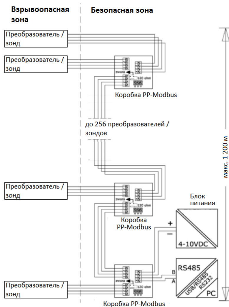
Рисунок 4 – Схема подключений электрическая исполнения Ex
